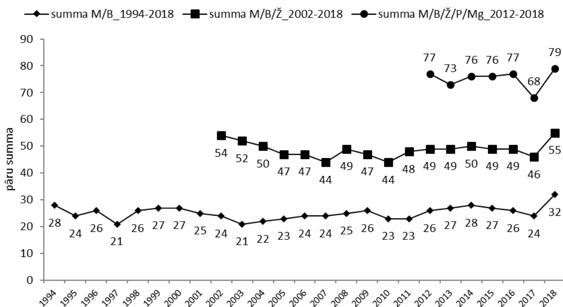
33. attēls. Mazo ērgļu skaita dinamika dažādos periodos, parauglaukumos ar nemainīgu platību
